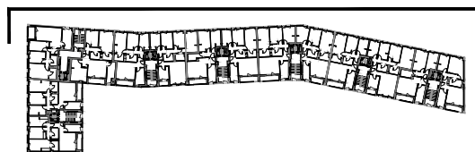
Edificio de 73 VPPA "Rosilla 02" - alzado norte
