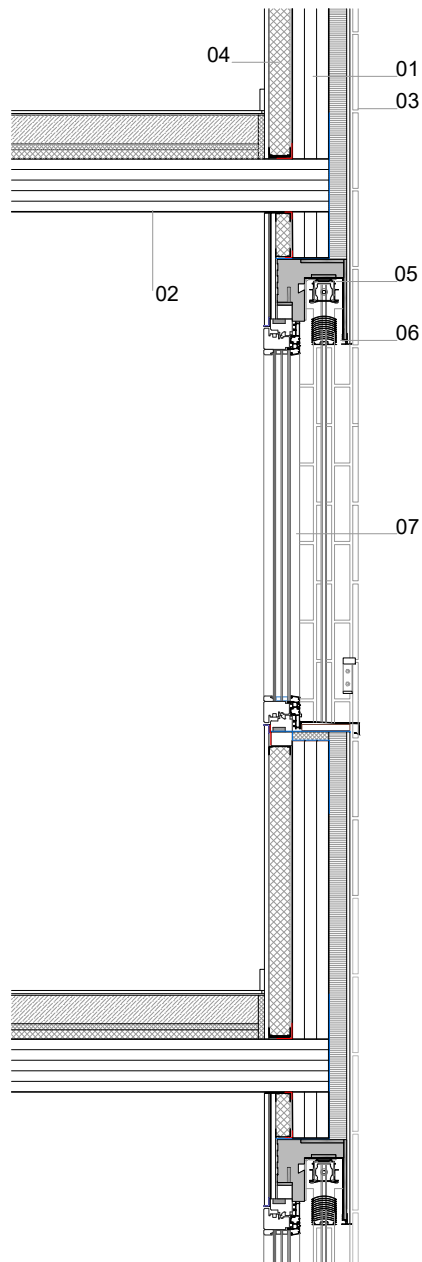
Sección transversal
