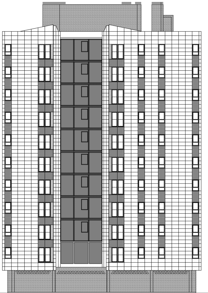
FACHADA SURESTE
