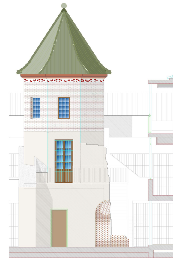
ALZADO OESTE
