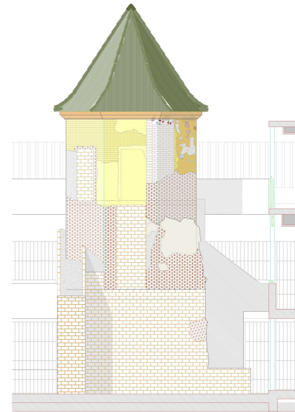
ALZADO OESTE
