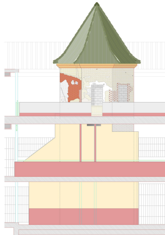
ALZADO ESTE
