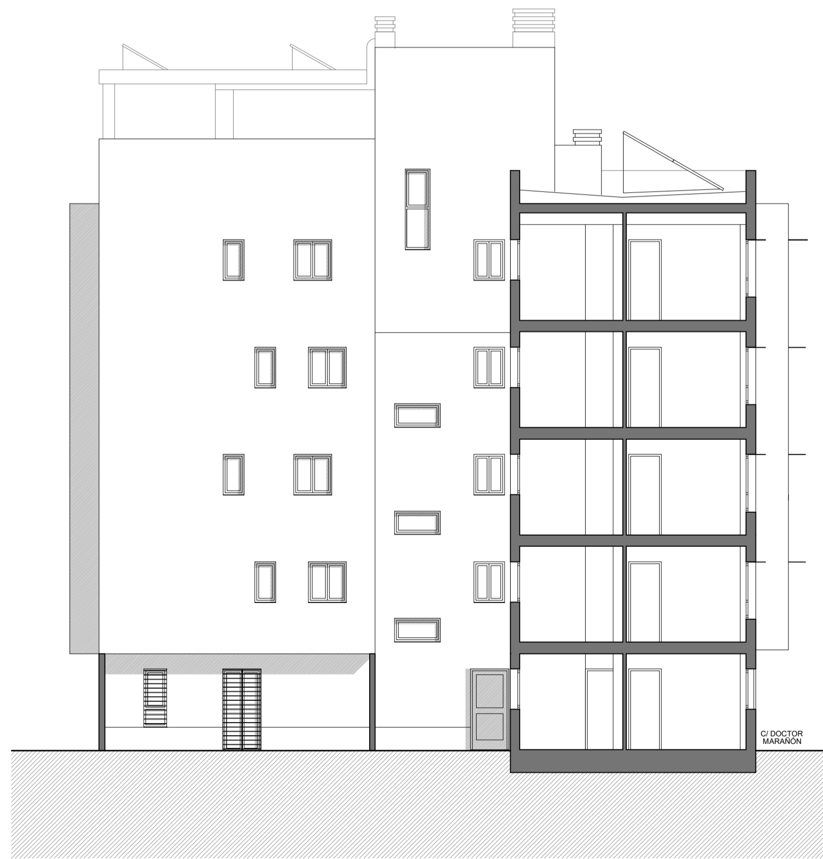
SECCIÓN E-E
