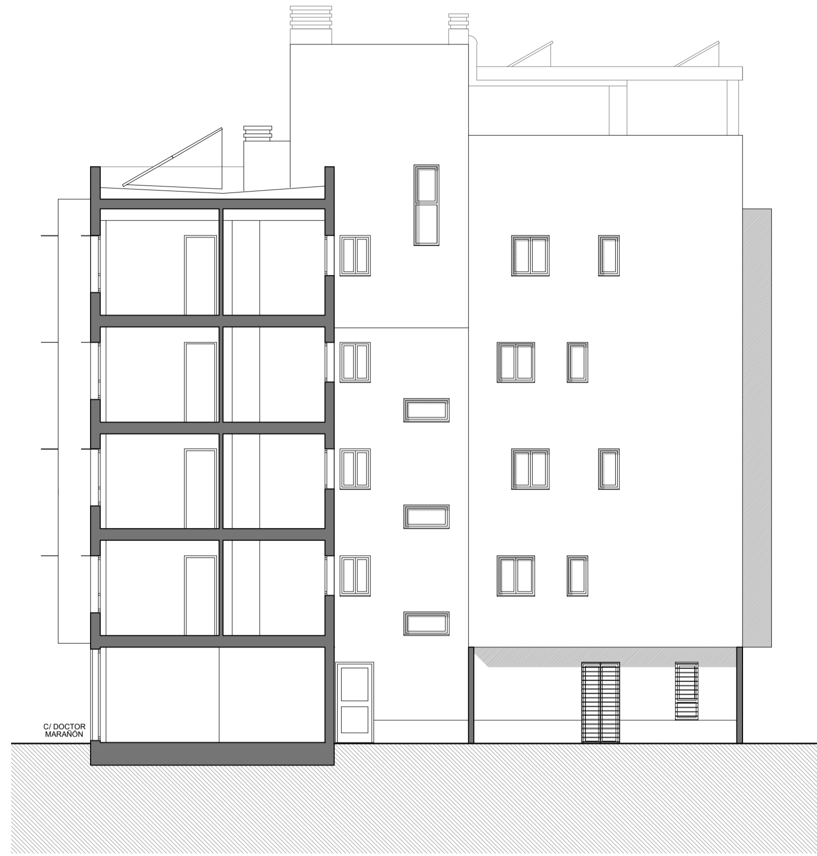
SECCIÓN C-C
