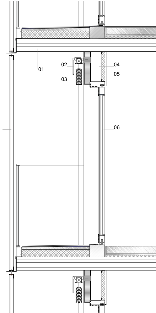
Sección transversal
