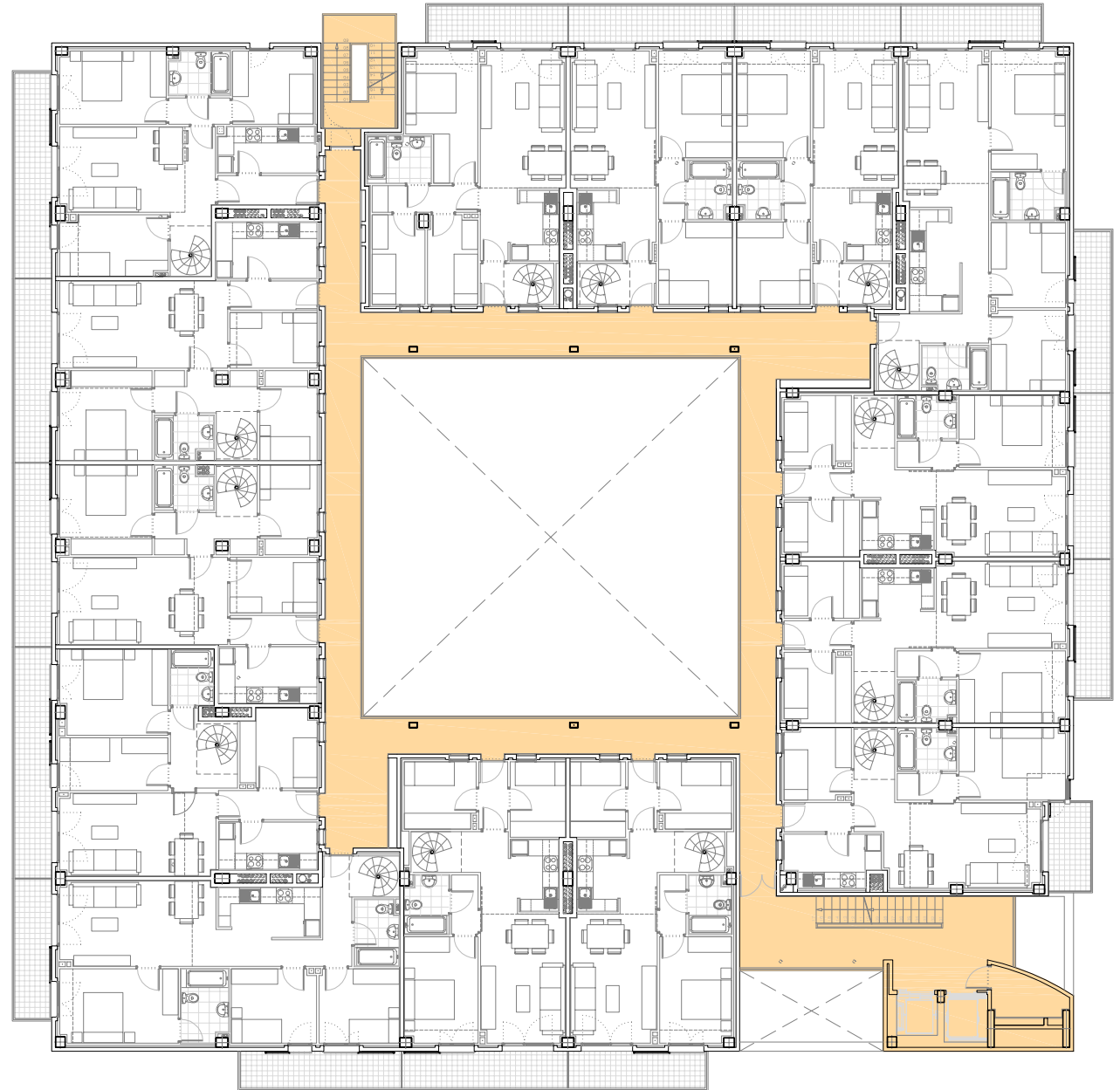
Planta sexta
