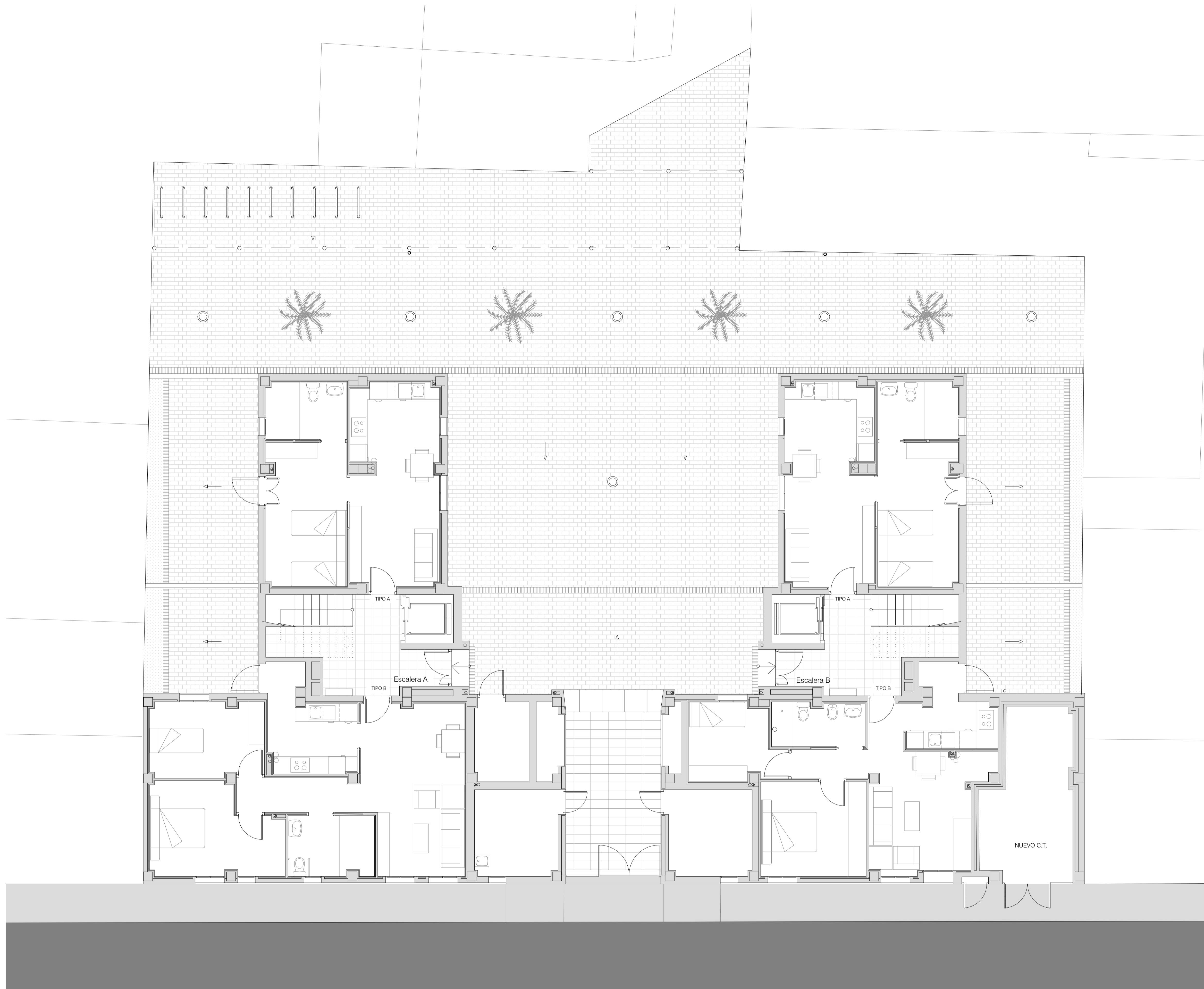
PLANTA BAJA Y PATIO DE PARCELA
