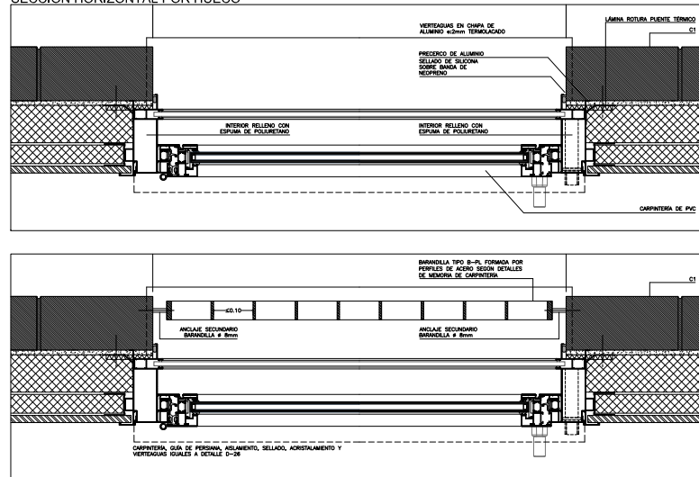
SECCIÓN HORIZONTAL POR HUECO
