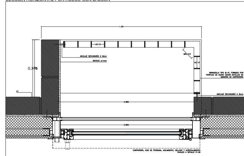
SECCIÓN HORIZONTAL POR HUECO CON BALCÓN
