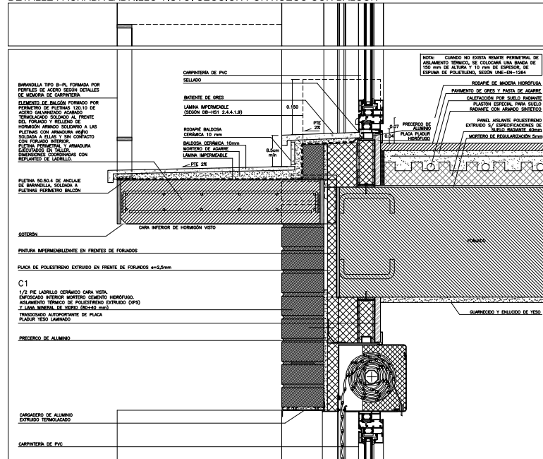
DETALLE FACHADA LADRILLO VISTO. SECCIÓN POR HUECO CON BALCÓN
