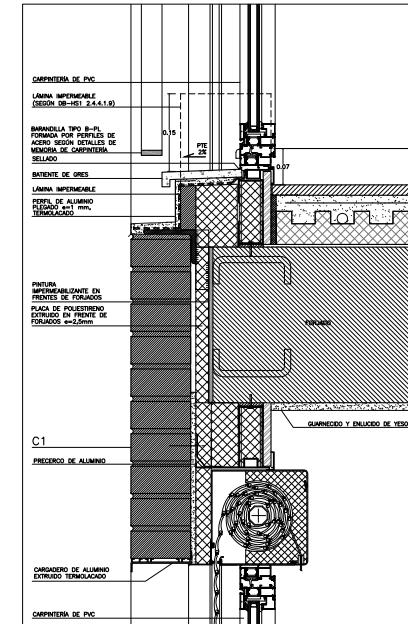
DETALLE FACHADA LADRILLO VISTO. SECCIÓN POR HUECO
