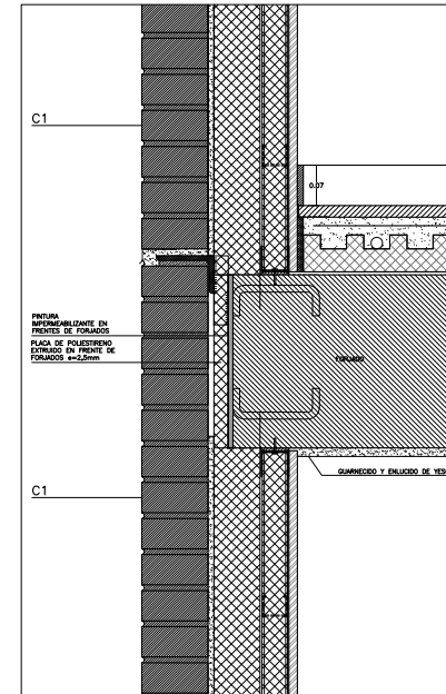
DETALLE FACHADA LADRILLO VISTO
